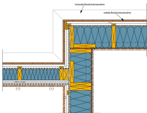
Anschluss Brüstung Terrasse an Aussenwand
